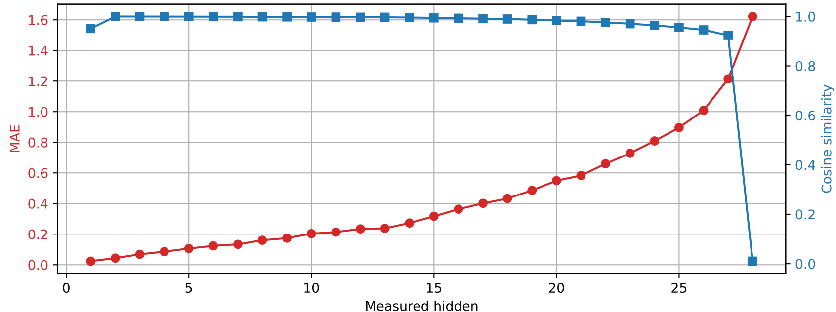
Llama-3.2-3B | Prompt 3 Spared layer 1 | Unquantized vs hybrid
