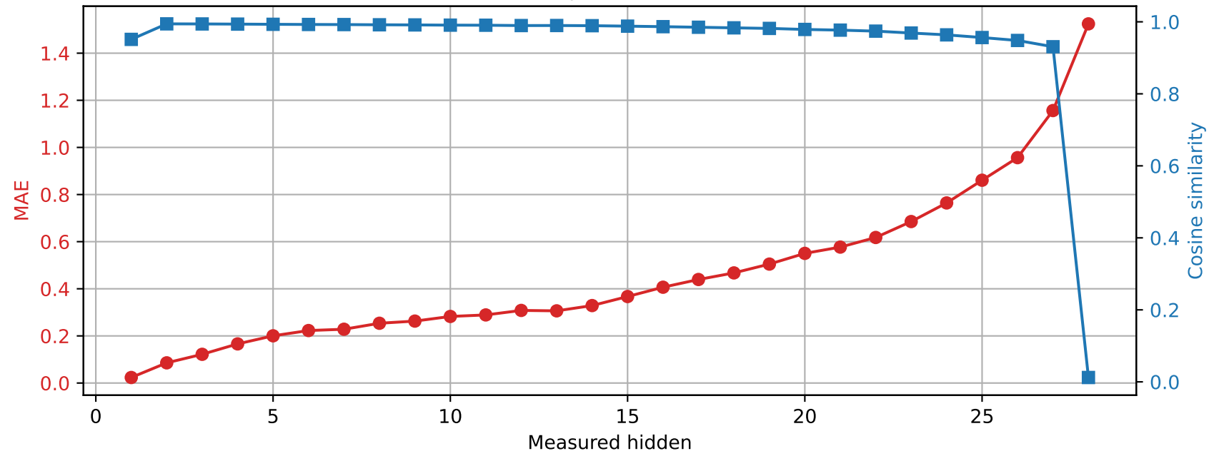
Llama-3.2-3B | Prompt 3 Spared layer 21 | Unquantized vs hybrid
