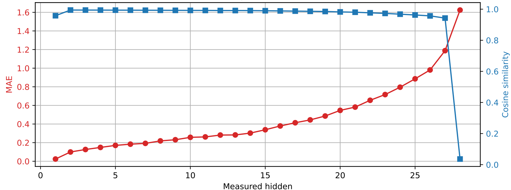
Llama-3.2-3B | Prompt 4 Spared layer 13 | Unquantized vs hybrid
