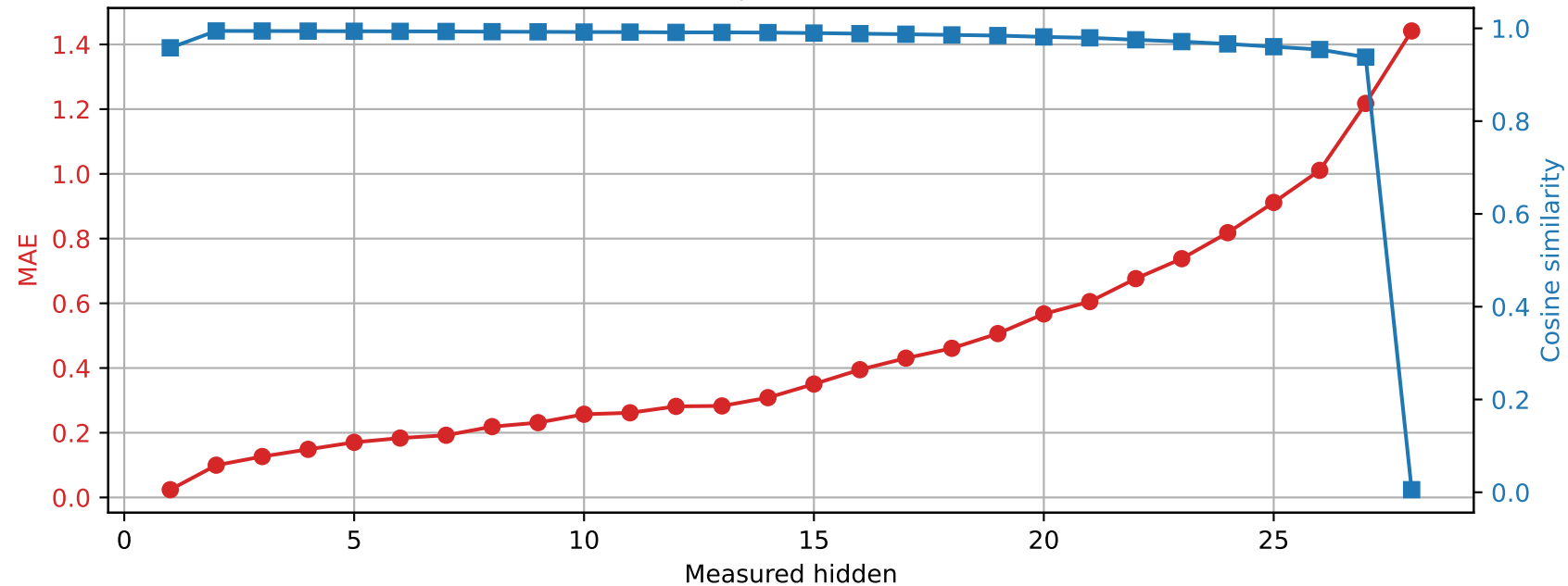
Llama-3.2-3B | Prompt 4 Spared layer 26 | Unquantized vs hybrid
