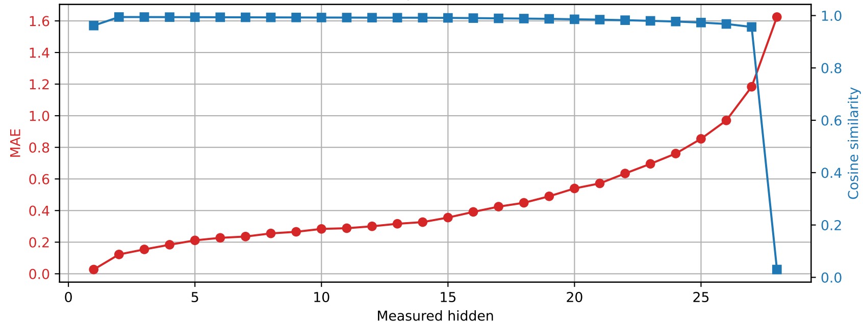
Llama-3.2-3B | Prompt 0 Spared layer 12 | Unquantized vs hybrid
