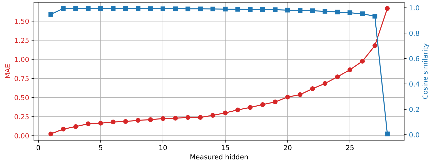
Llama-3.2-3B | Prompt 1 Spared layer 4 | Unquantized vs hybrid
