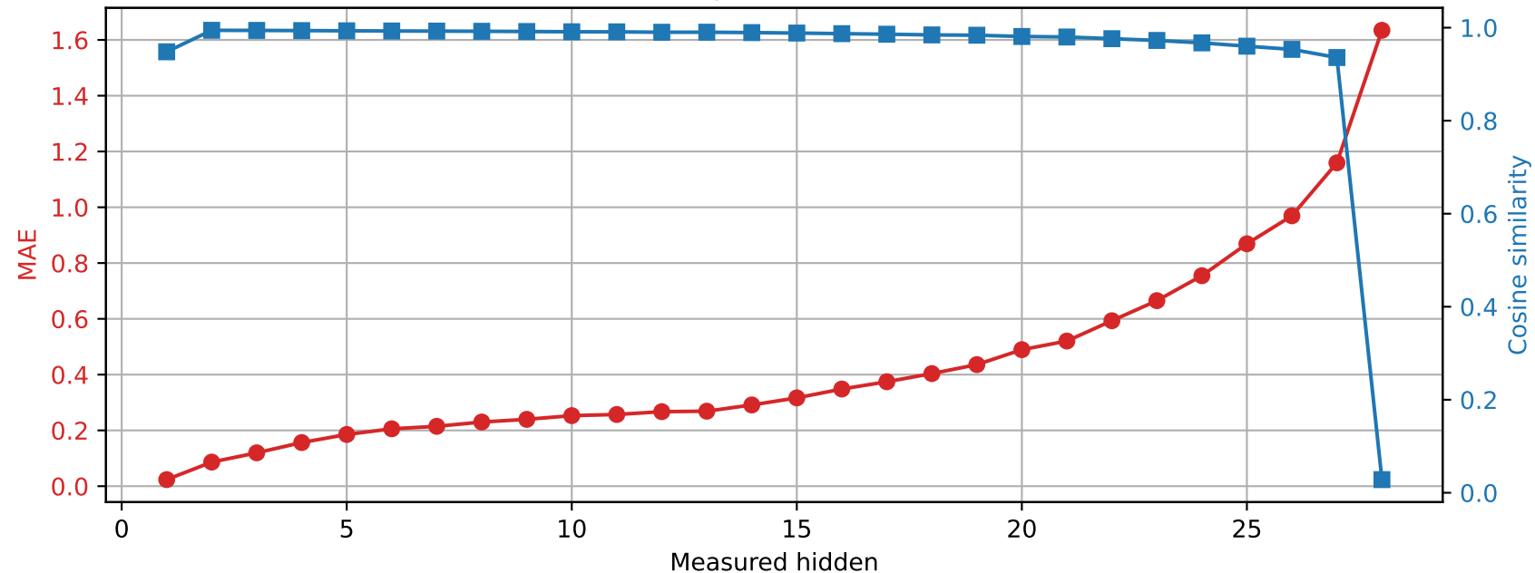
Llama-3.2-3B | Prompt 1 Spared layer 6 | Unquantized vs hybrid
