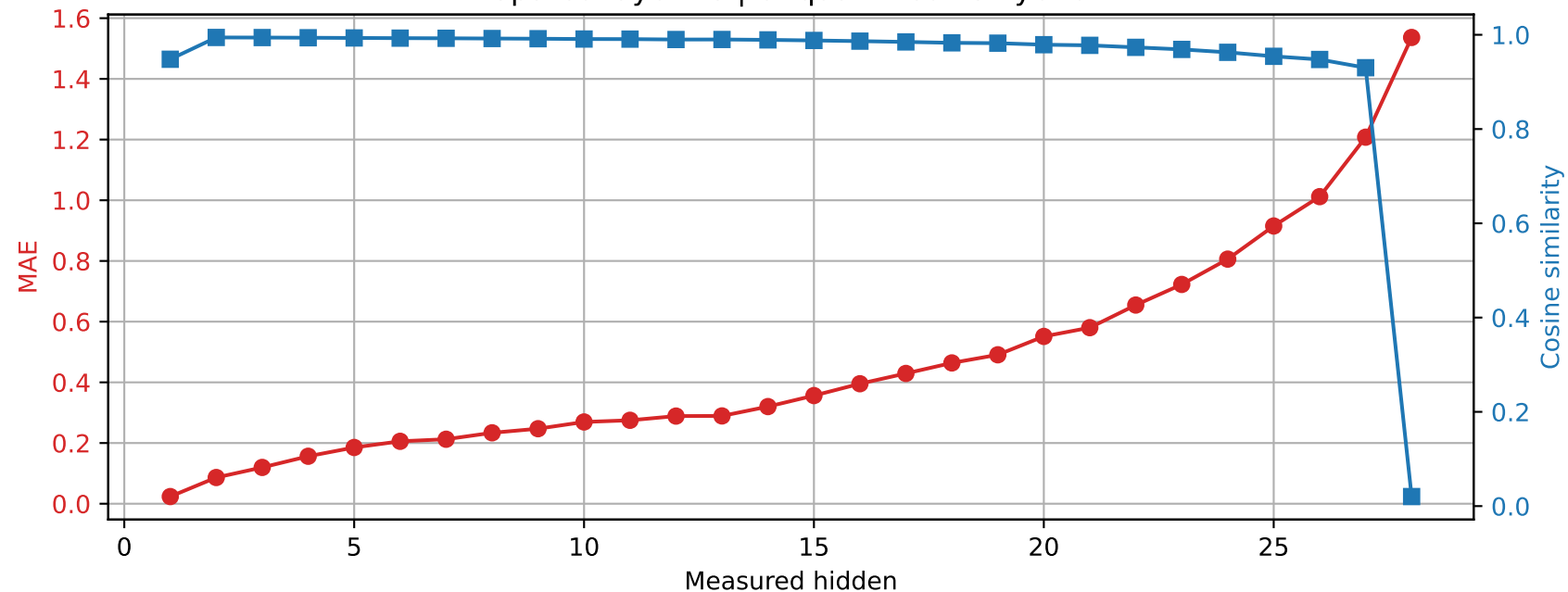
Llama-3.2-3B | Prompt 1 Spared layer 10 | Unquantized vs hybrid
