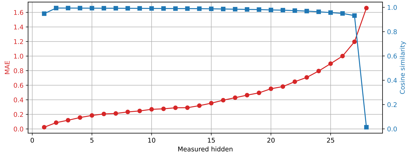
Llama-3.2-3B | Prompt 1 Spared layer 18 | Unquantized vs hybrid
