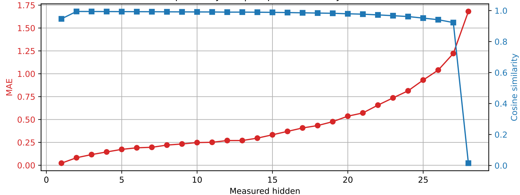
Llama-3.2-3B | Prompt 2 Spared layer 9 | Unquantized vs hybrid
