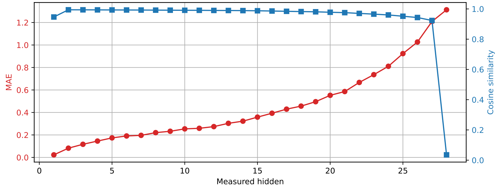
Llama-3.2-3B | Prompt 2 Spared layer 12 | Unquantized vs hybrid
