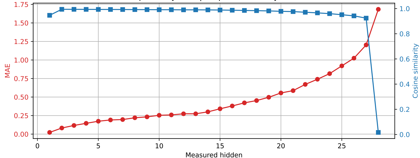
Llama-3.2-3B | Prompt 2 Spared layer 19 | Unquantized vs hybrid
