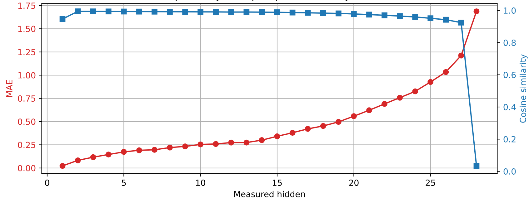
Llama-3.2-3B | Prompt 2 Spared layer 20 | Unquantized vs hybrid
