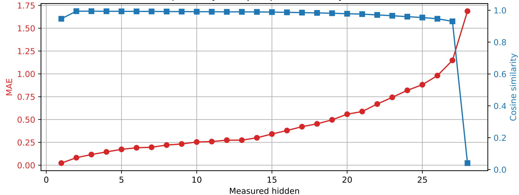
Llama-3.2-3B | Prompt 2 Spared layer 24 | Unquantized vs hybrid
