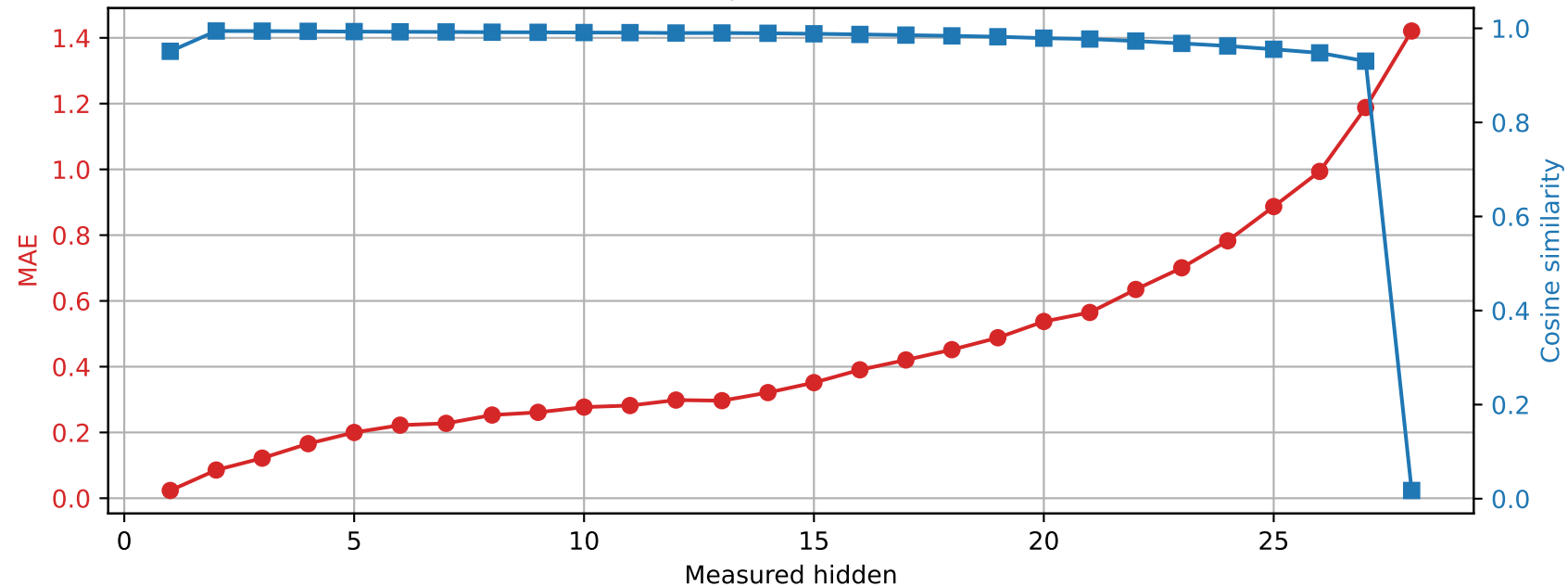
Llama-3.2-3B | Prompt 3 Spared layer 8 | Unquantized vs hybrid
