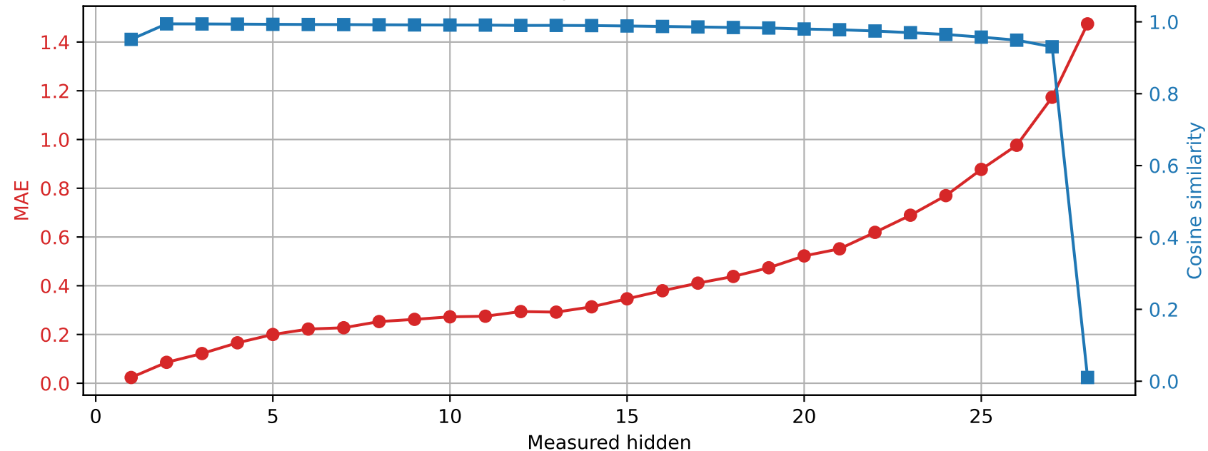
Llama-3.2-3B | Prompt 3 Spared layer 9 | Unquantized vs hybrid
