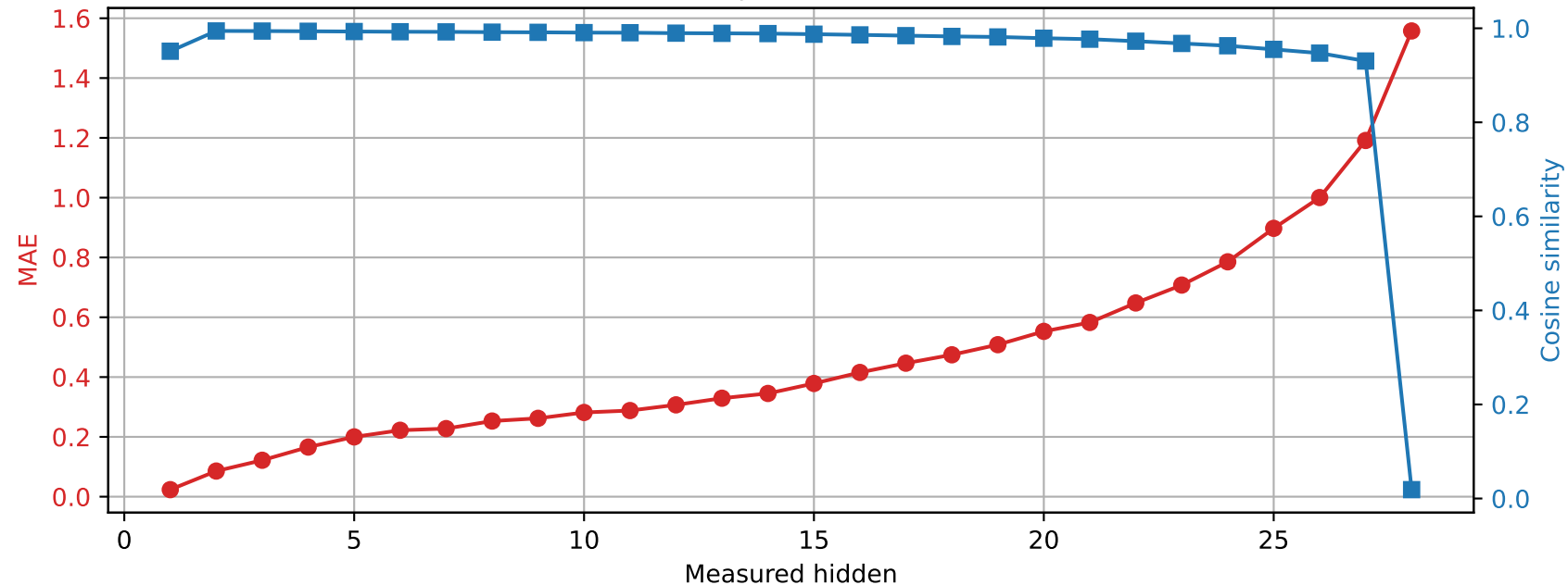
Llama-3.2-3B | Prompt 3 Spared layer 12 | Unquantized vs hybrid
