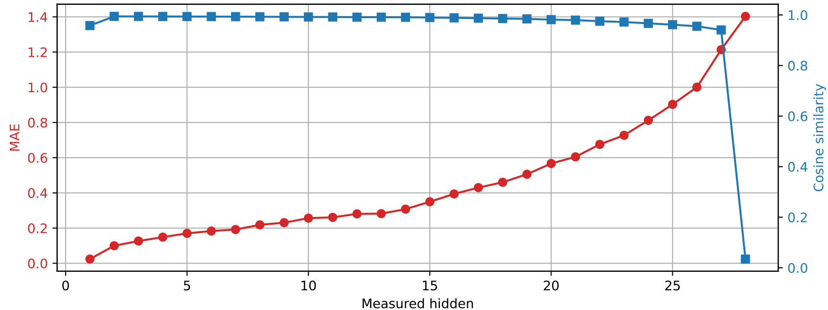
Llama-3.2-3B | Prompt 4 Spared layer 22 | Unquantized vs hybrid
