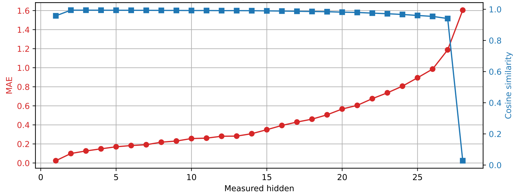
Llama-3.2-3B | Prompt 4 Spared layer 23 | Unquantized vs hybrid
