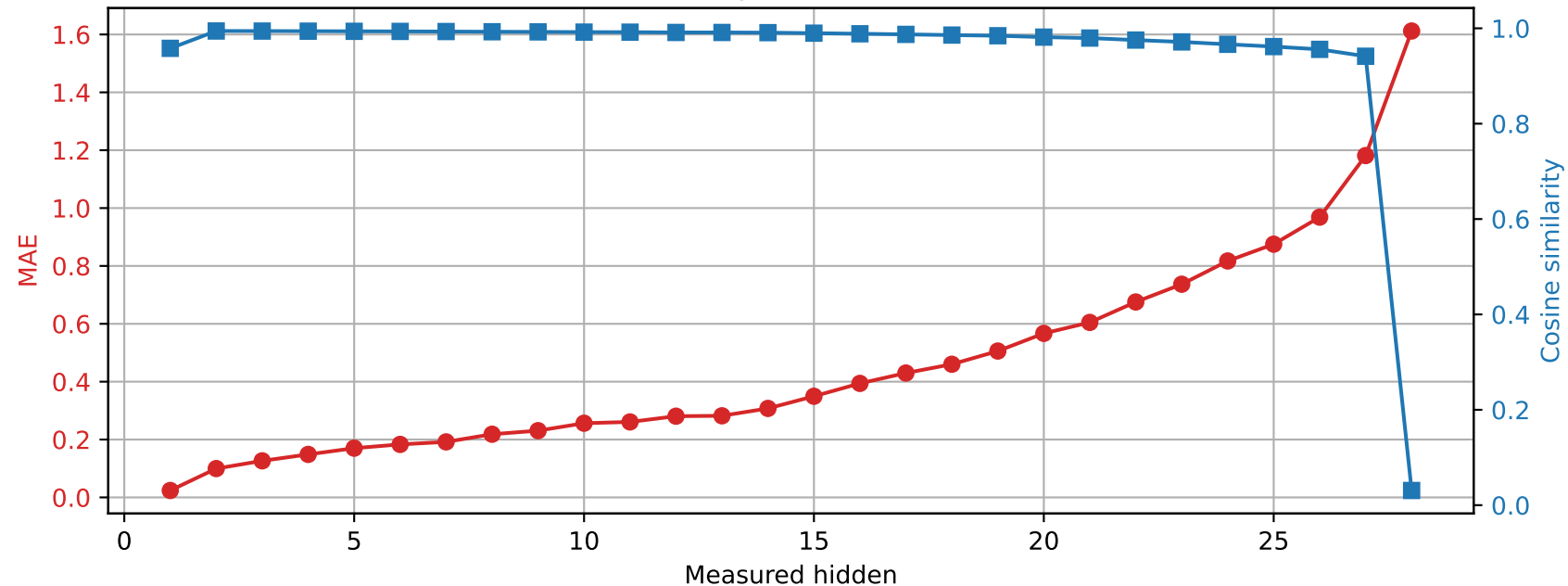
Llama-3.2-3B | Prompt 4 Spared layer 24 | Unquantized vs hybrid
