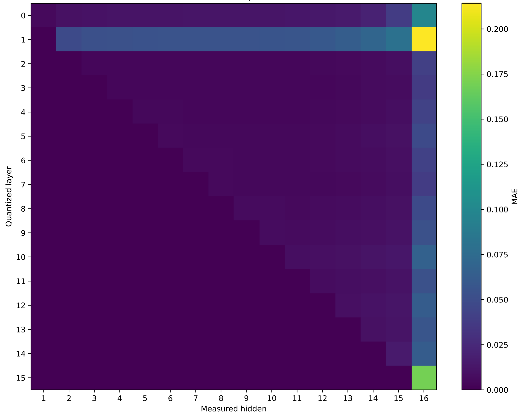
Model: Llama-3.2-1B | float16 \rightarrow int8
