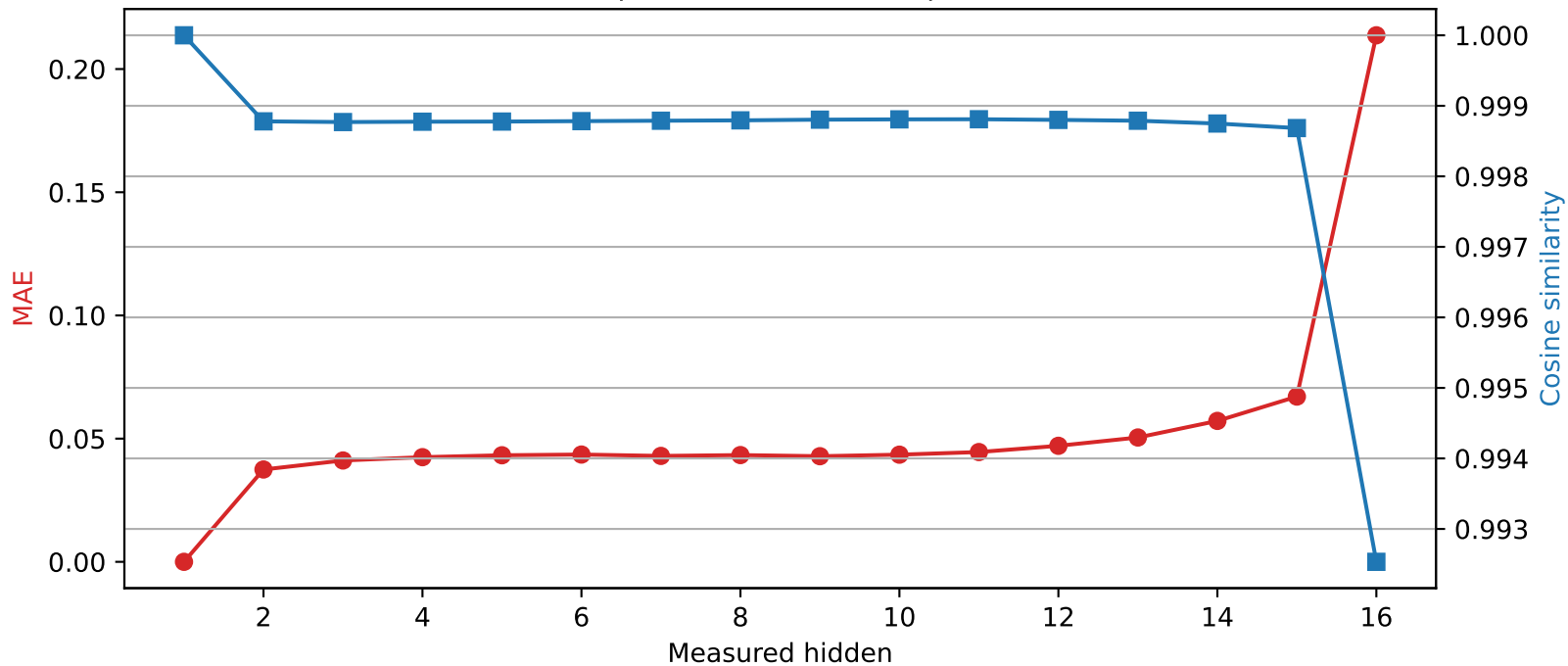
Llama-3.2-1B | Quantized layer 1 | float16 \rightarrow int8
