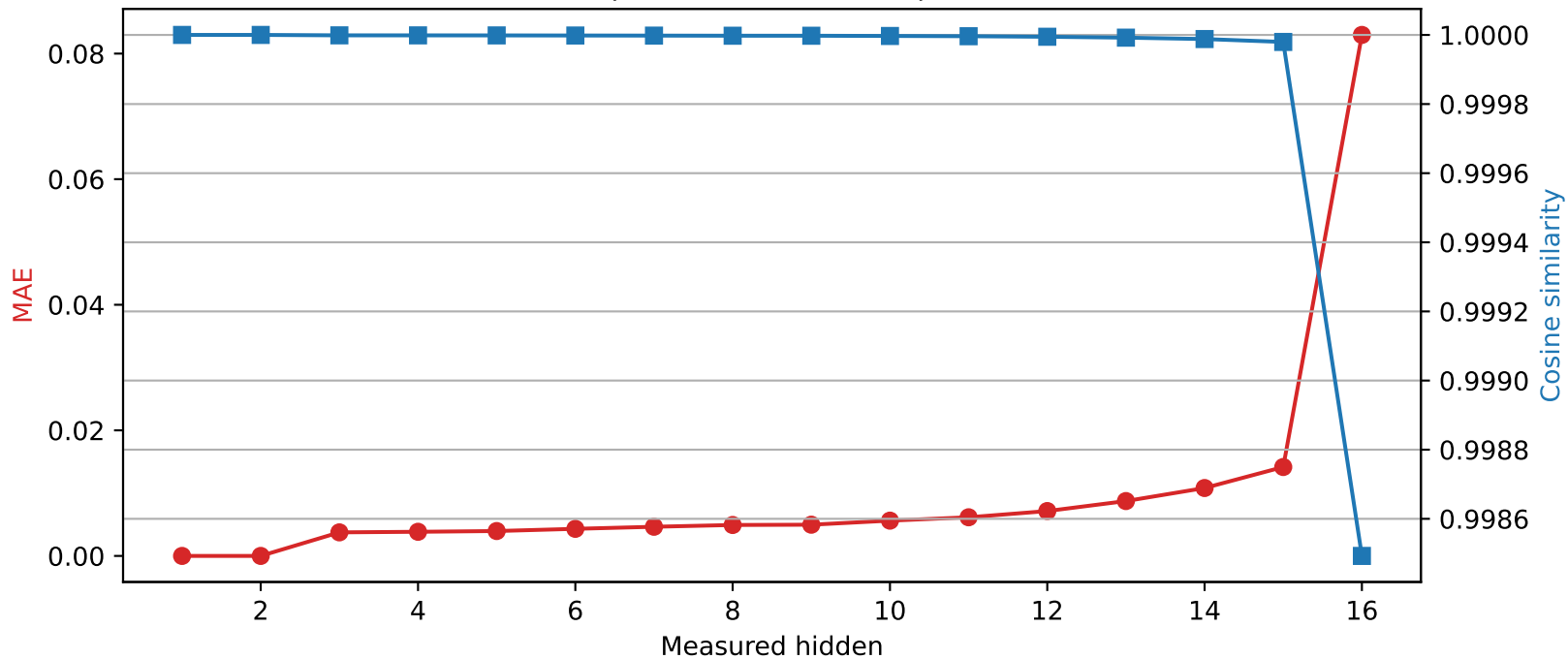
Llama-3.2-1B | Quantized layer 2 | float16 \rightarrow int8
