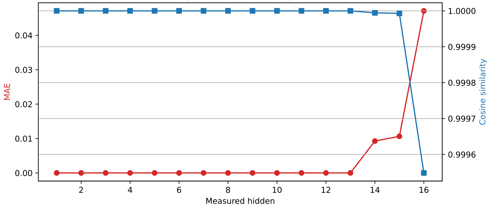
Llama-3.2-1B | Quantized layer 13 | float32 \rightarrow int8
