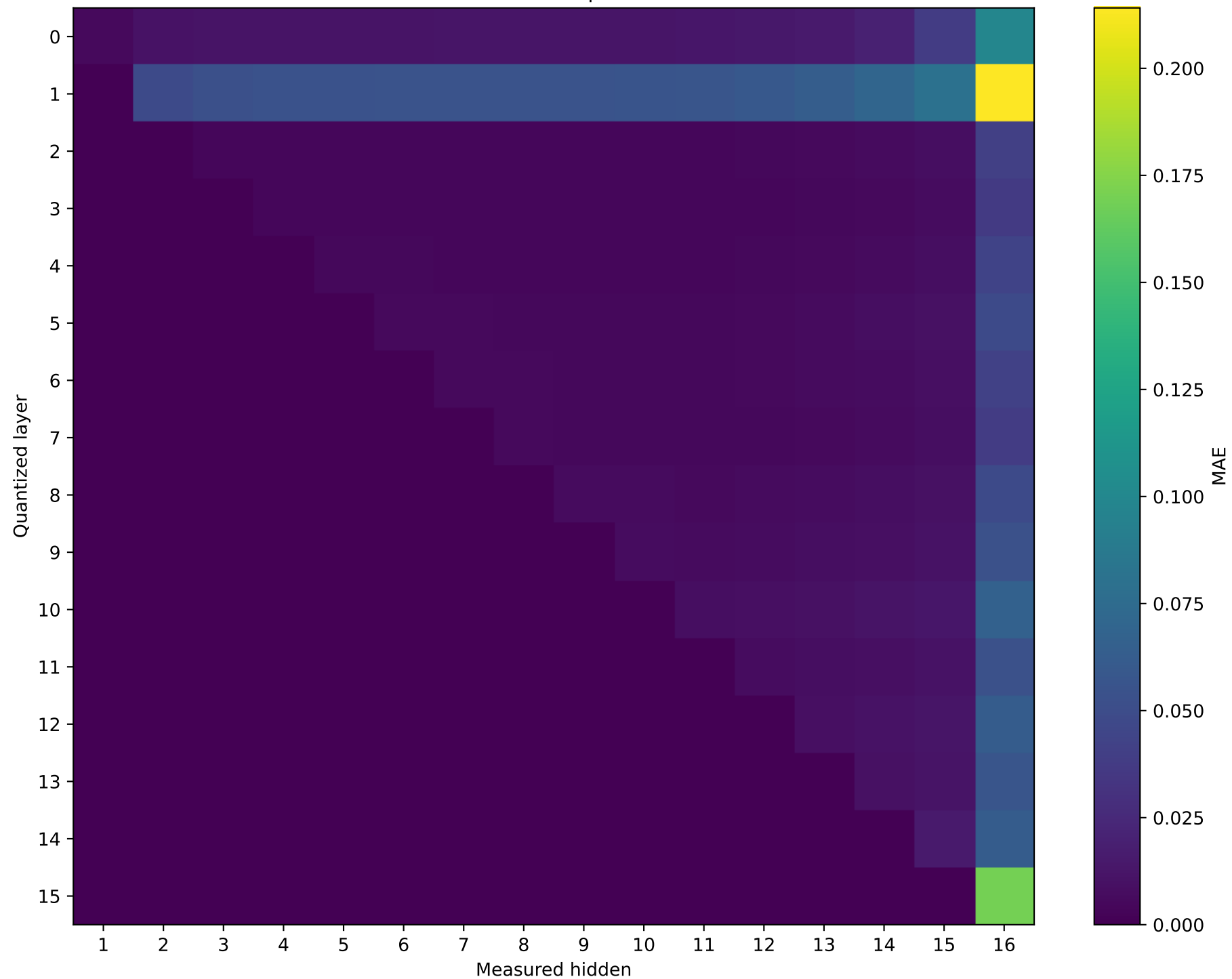
Model: Llama-3.2-1B | float64 → int8
