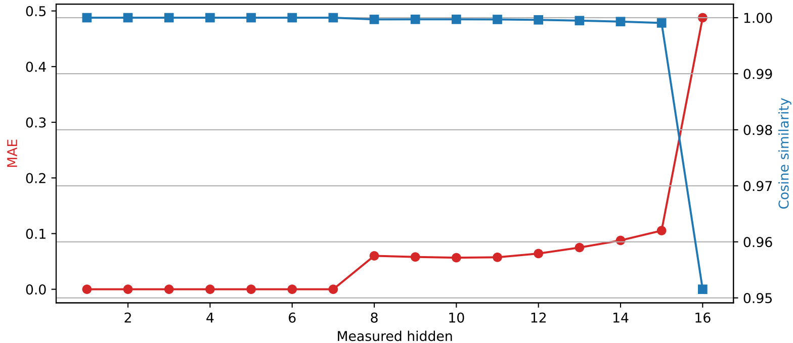
Llama-3.2-1B | Quantized layer 7 | float16 \rightarrow int4
