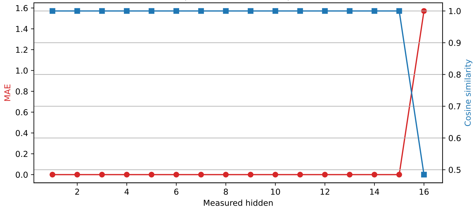
Llama-3.2-1B | Quantized layer 15 | float16 \rightarrow int4
