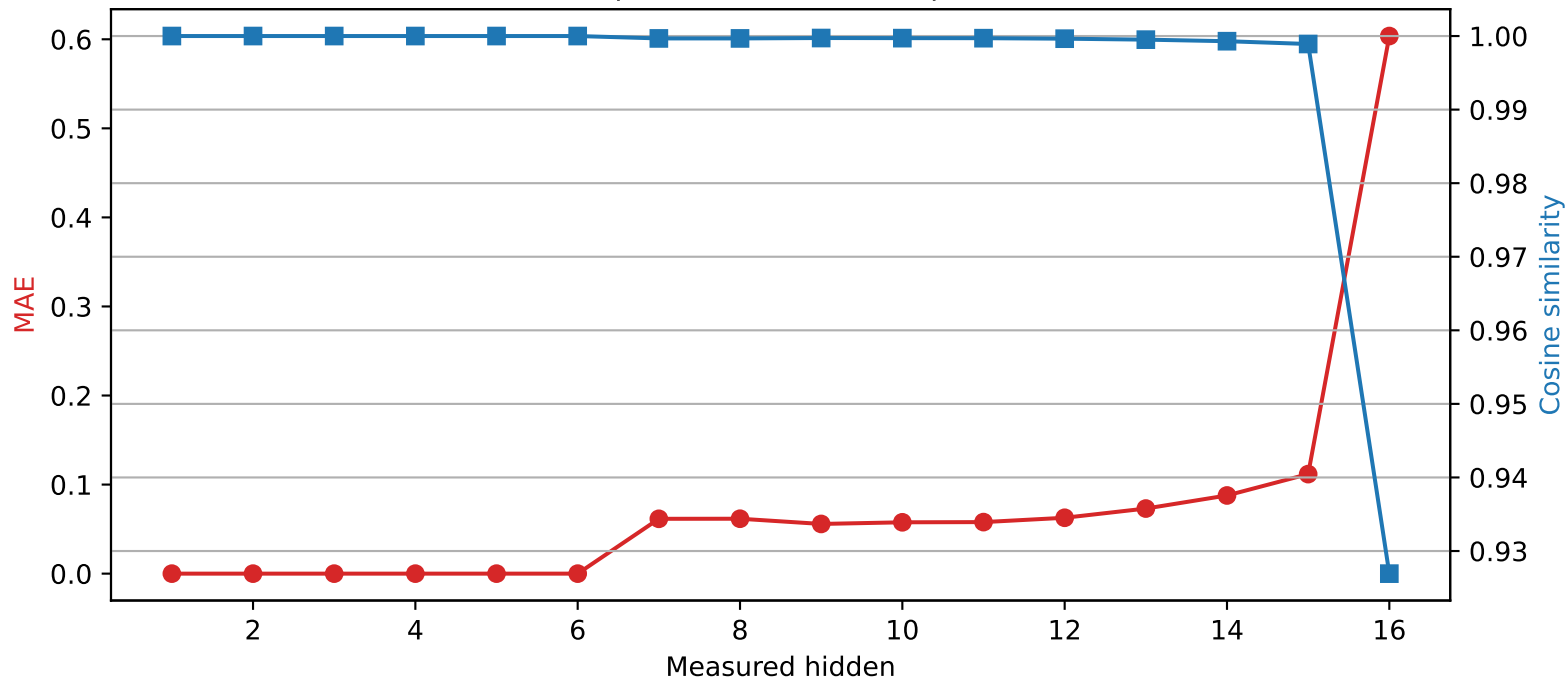
Llama-3.2-1B | Quantized layer 6 | float16 \rightarrow int4
