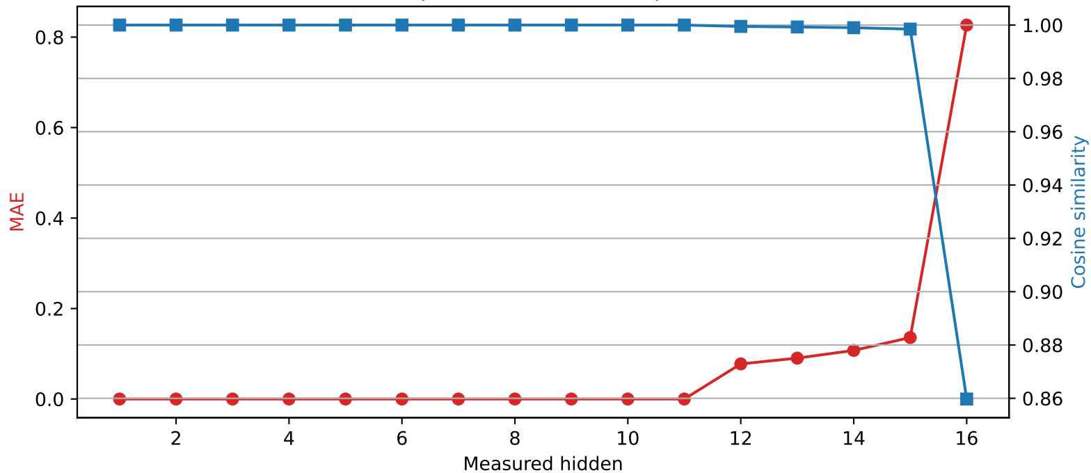
Llama-3.2-1B | Quantized layer 11 | float16 \rightarrow int4
