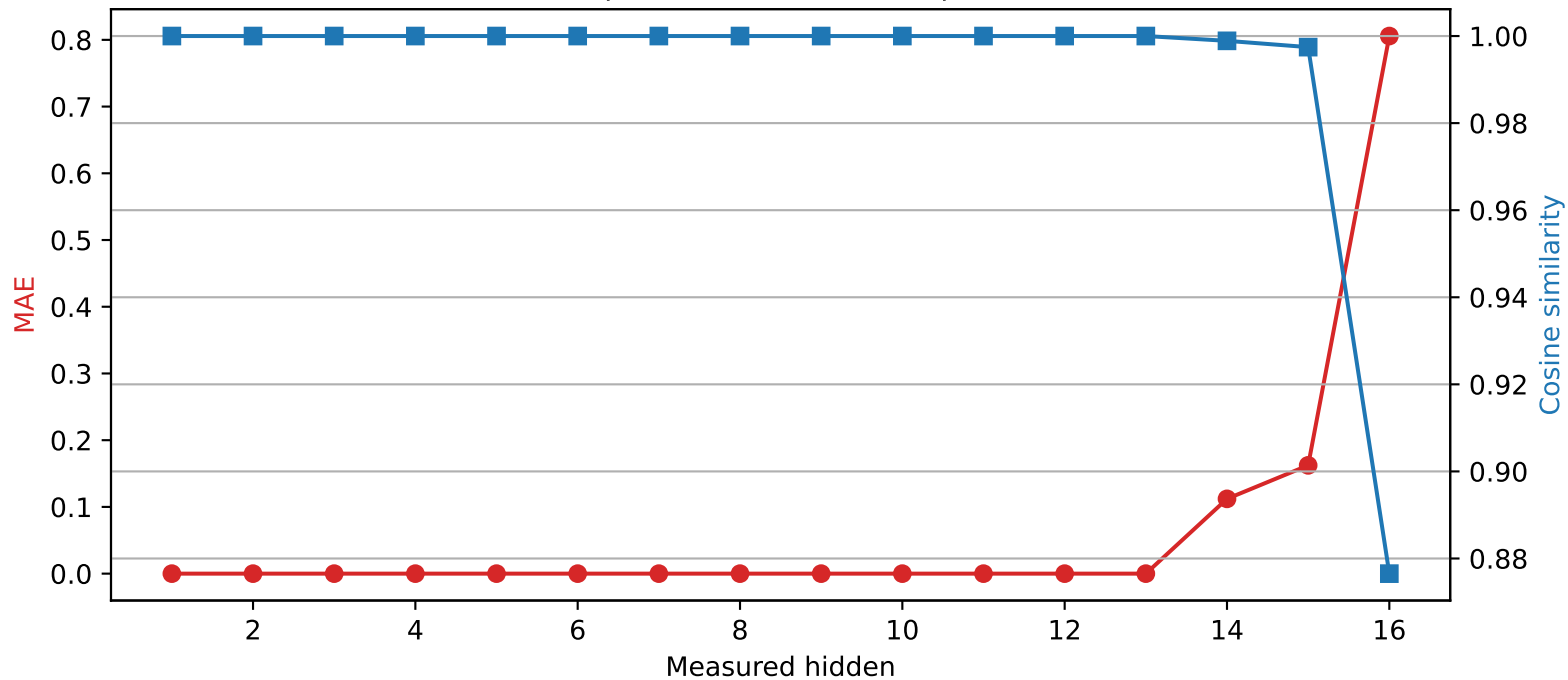
Llama-3.2-1B | Quantized layer 13 | float16 \rightarrow int4
