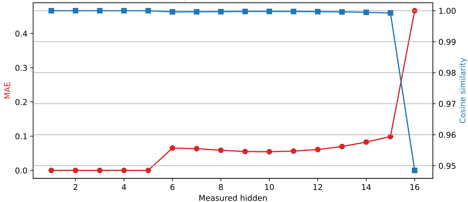
Llama-3.2-1B | Quantized layer 5 | float16 \rightarrow int4
