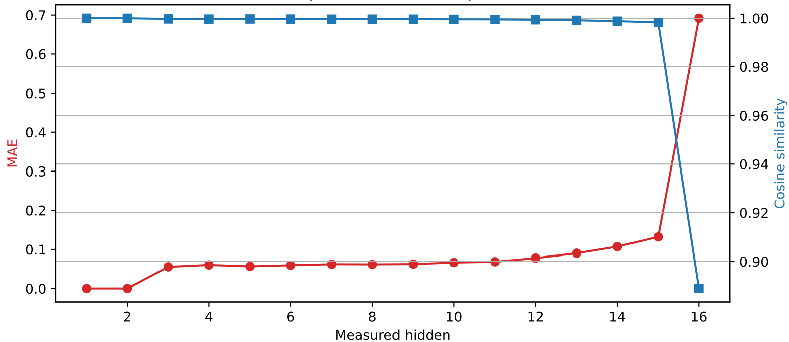
Llama-3.2-1B | Quantized layer 2 | float32 \rightarrow int4
