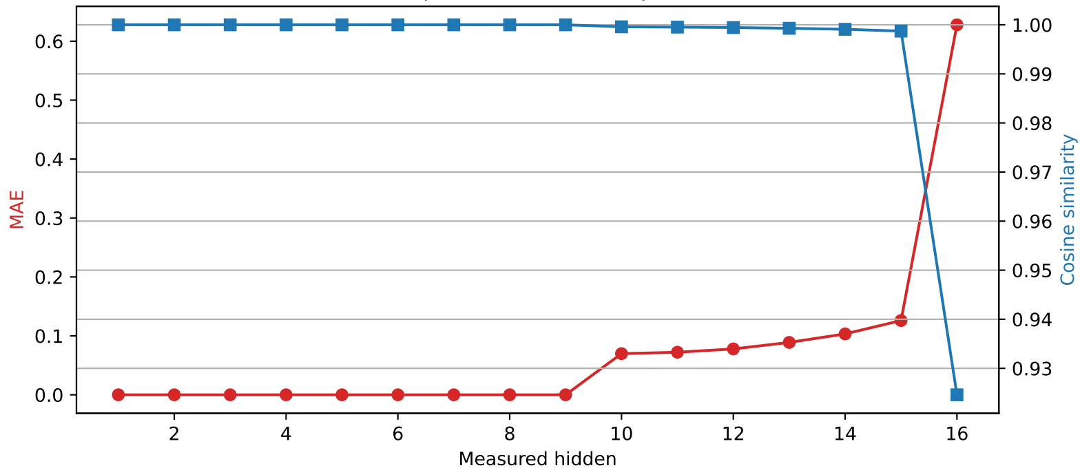
Llama-3.2-1B | Quantized layer 9 | float32 \rightarrow int4
