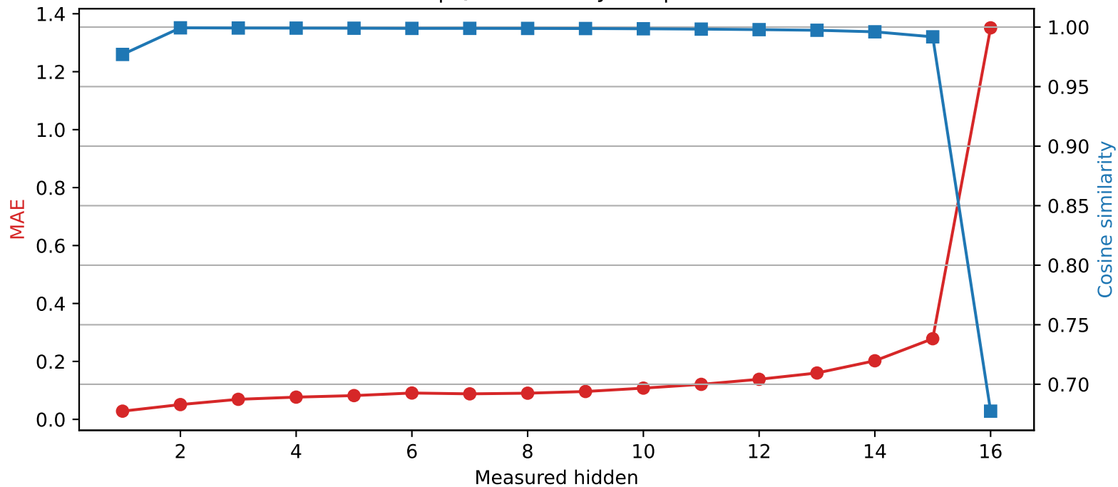
Llama-3.2-1B | Quantized layer 0 | float32 \rightarrow int4
