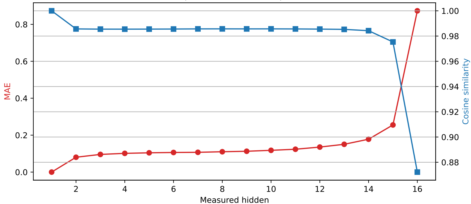
Llama-3.2-1B | Quantized layer 1 | float32 \rightarrow int4
