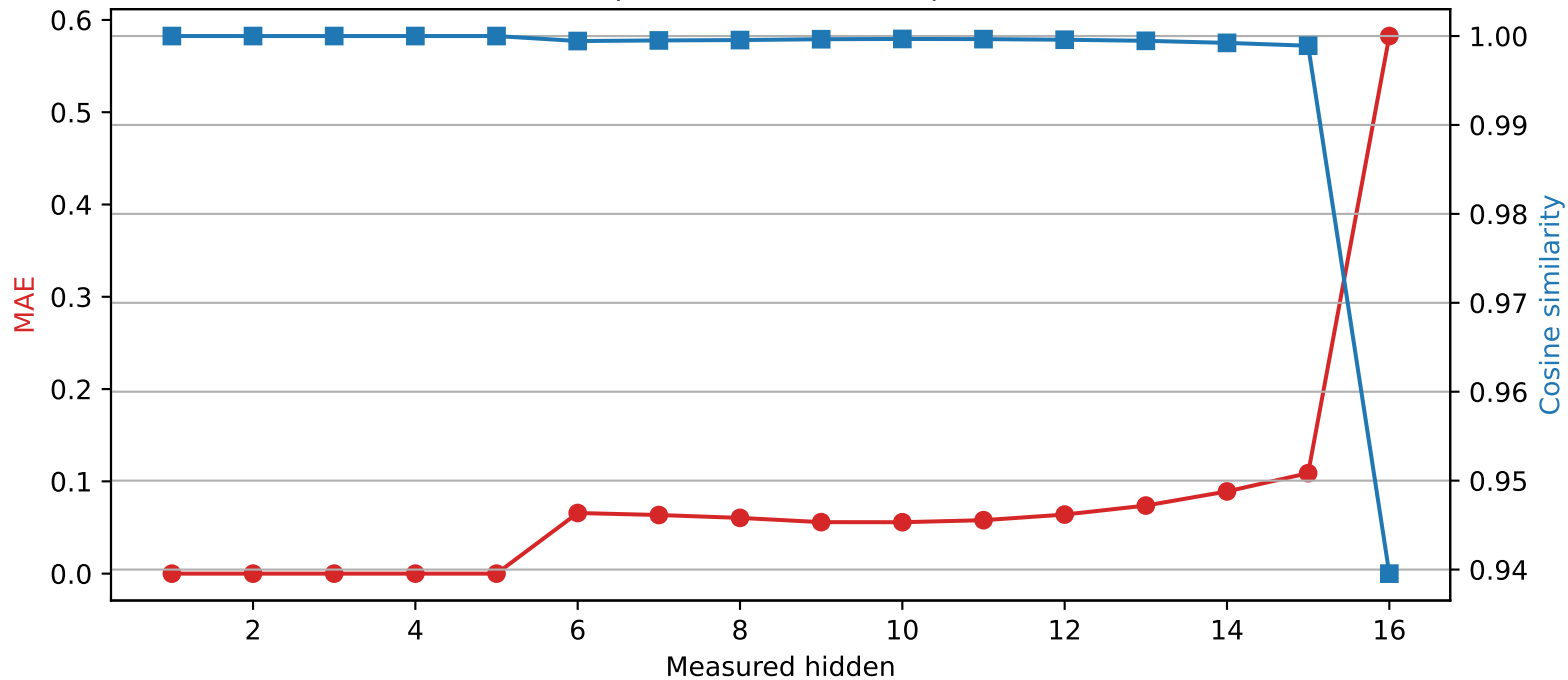
Llama-3.2-1B | Quantized layer 5 | float32 \rightarrow int4
