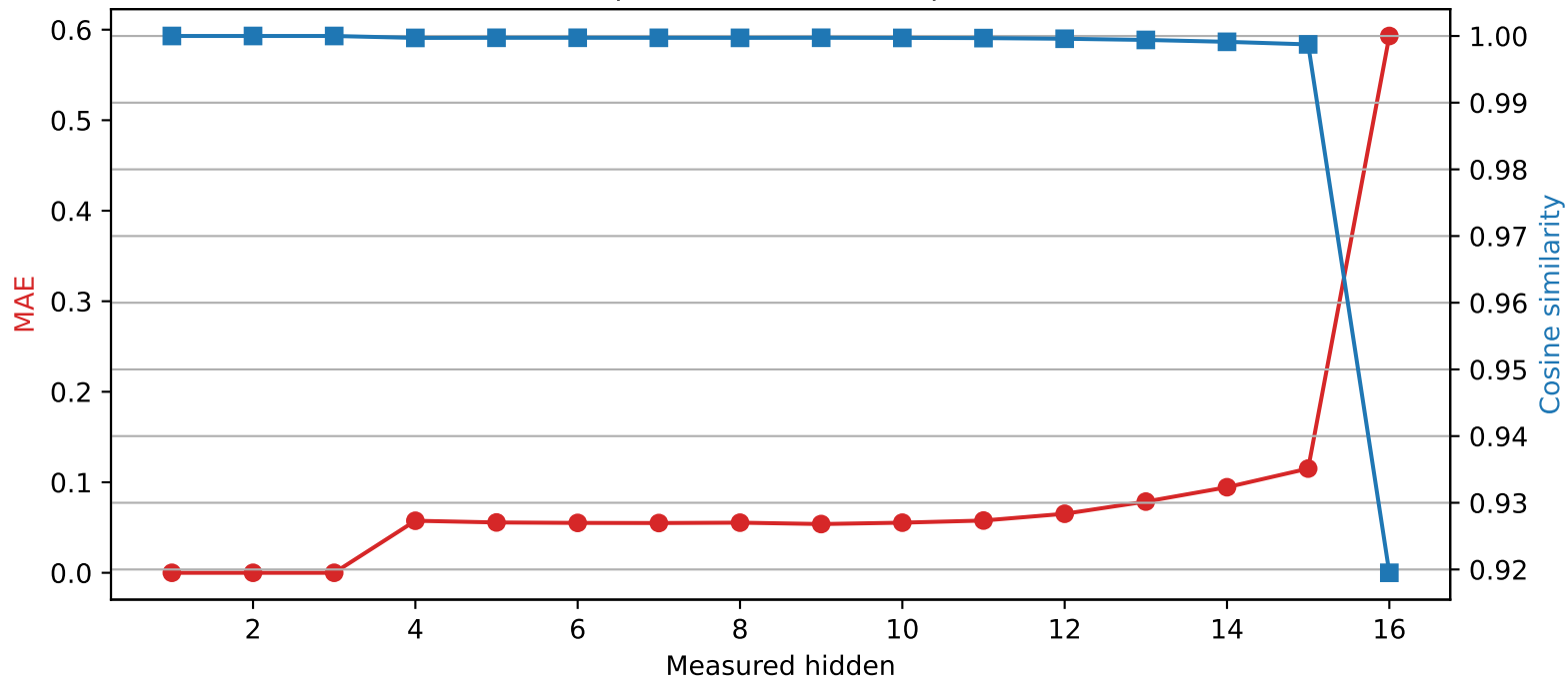
Llama-3.2-1B | Quantized layer 3 | float64 \rightarrow int4
