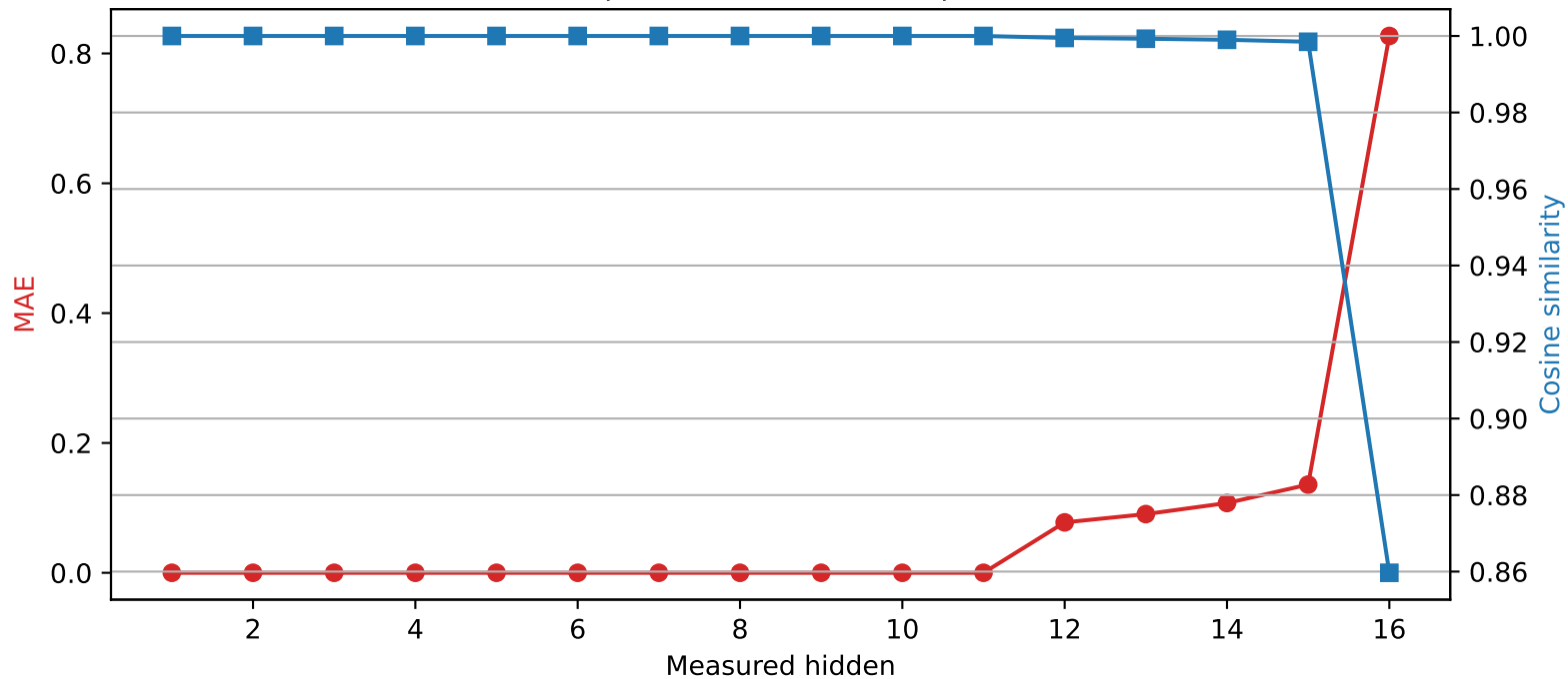
Llama-3.2-1B | Quantized layer 11 | float64 \rightarrow int4
