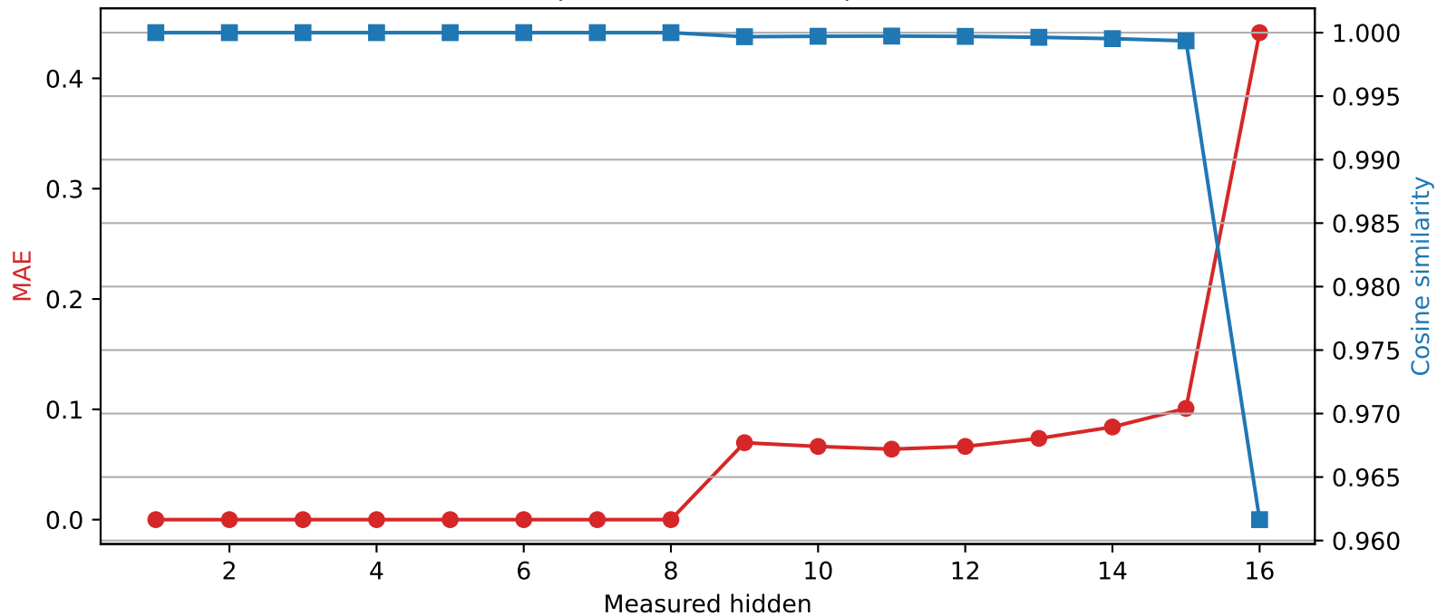
Llama-3.2-1B | Quantized layer 8 | float64 \rightarrow int4
