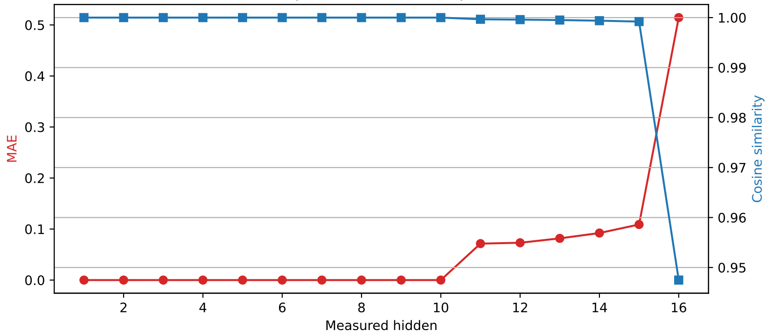
Llama-3.2-1B | Quantized layer 10 | float64 \rightarrow int4
