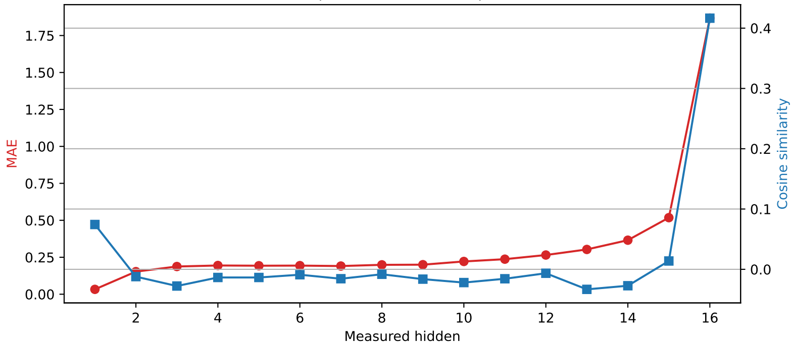
Llama-3.2-1B | Quantized layer 0 | float16 \rightarrow int2
