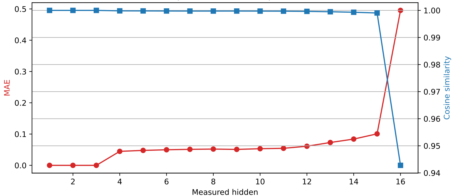
Llama-3.2-1B | Quantized layer 3 | float16 \rightarrow int2
