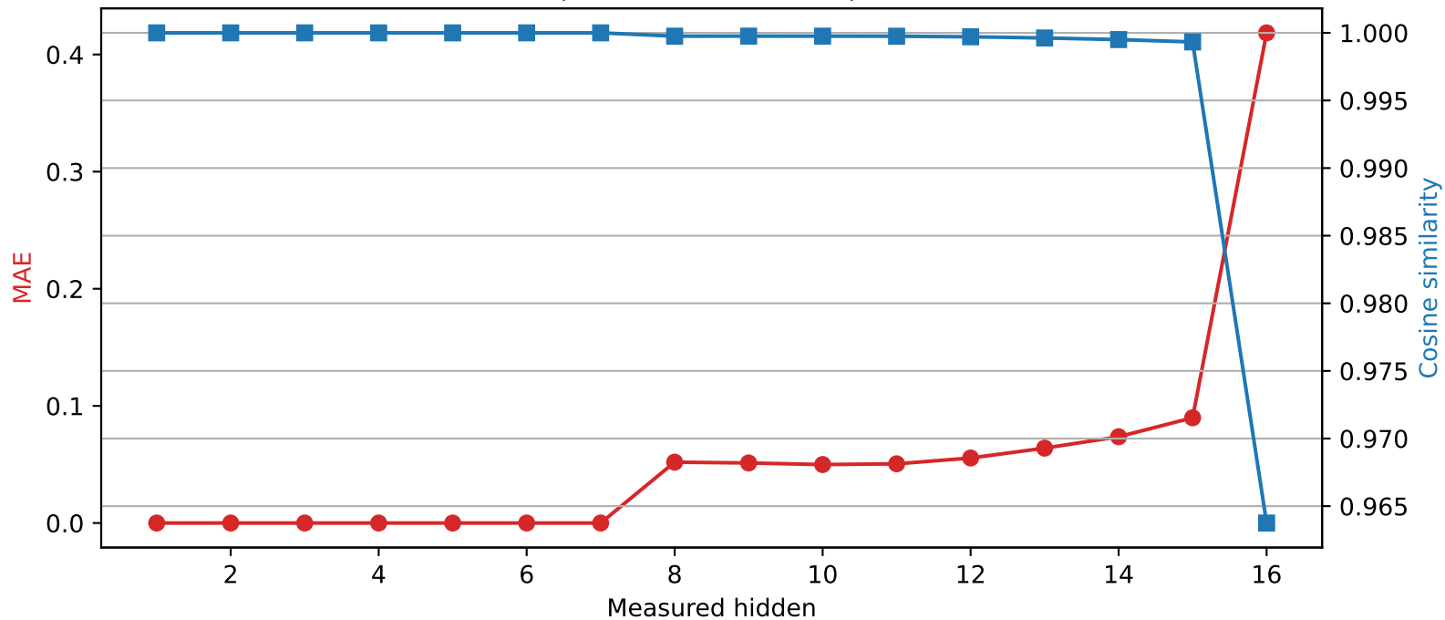
Llama-3.2-1B | Quantized layer 7 | float16 \rightarrow int2
