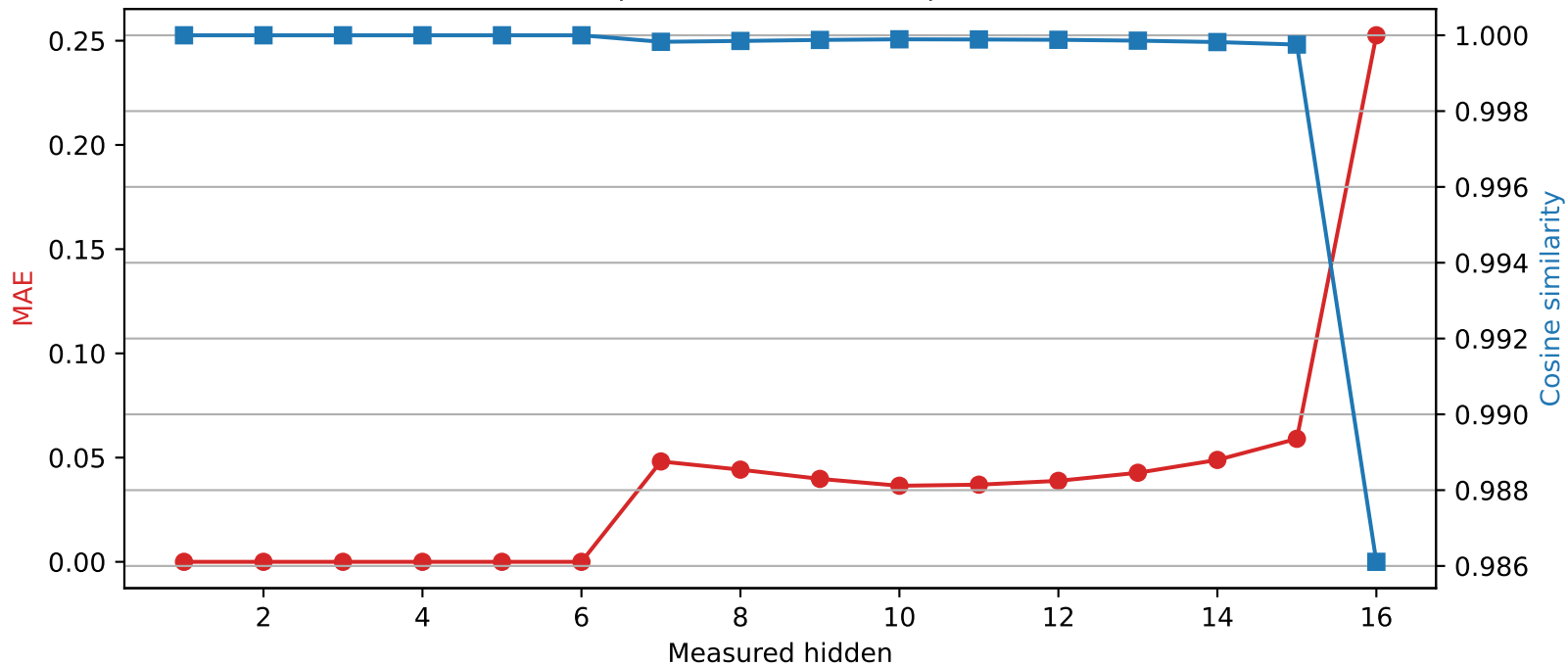
Llama-3.2-1B | Quantized layer 6 | float16 \rightarrow int2
