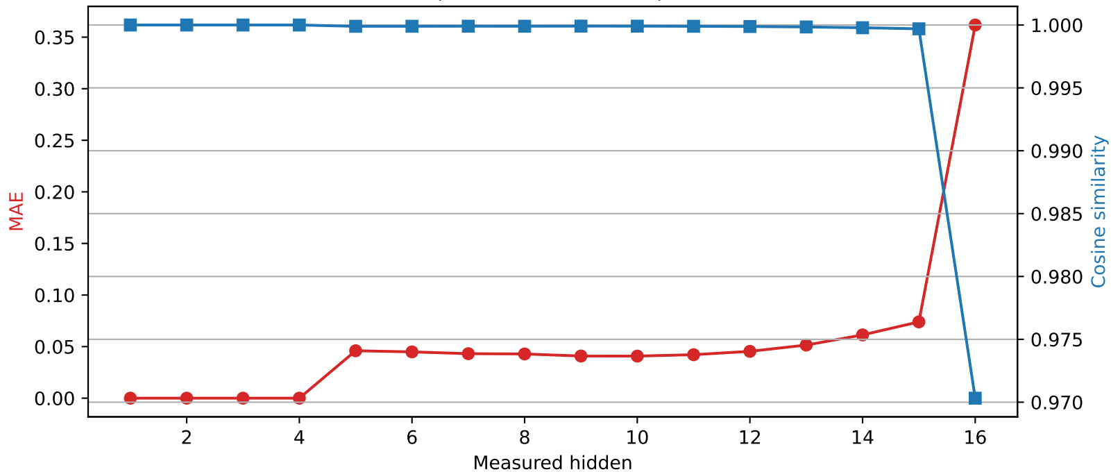
Llama-3.2-1B | Quantized layer 4 | float32 \rightarrow int2
