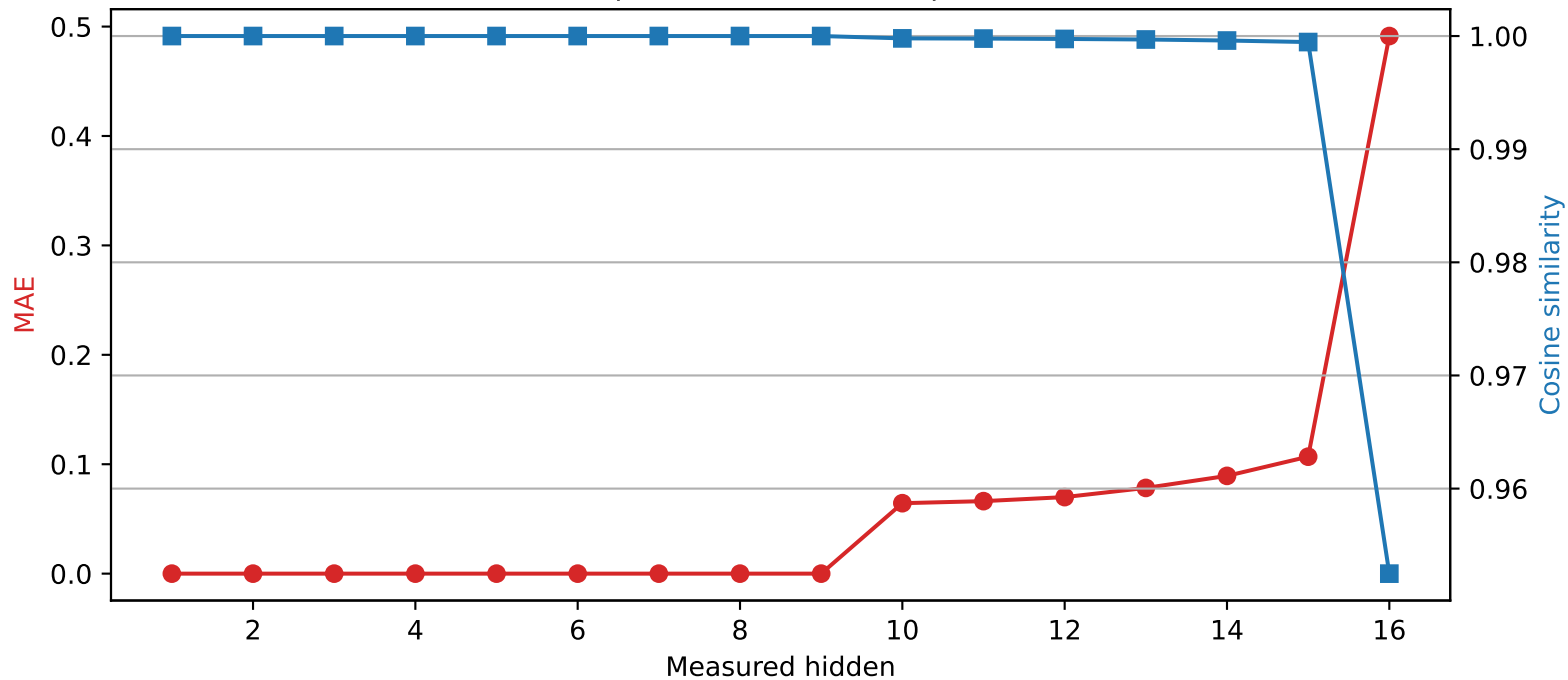
Llama-3.2-1B | Quantized layer 9 | float32 \rightarrow int2
