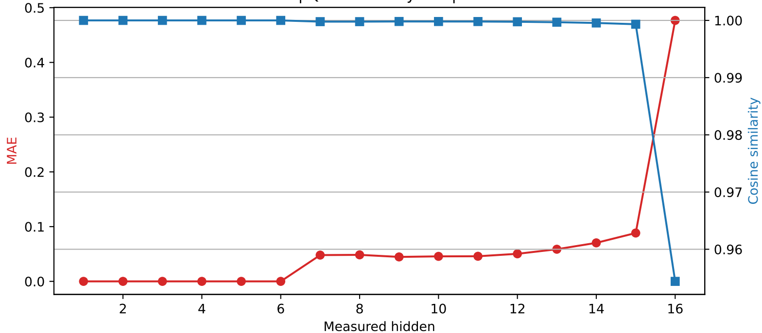
Llama-3.2-1B | Quantized layer 6 | float32 \rightarrow int2
