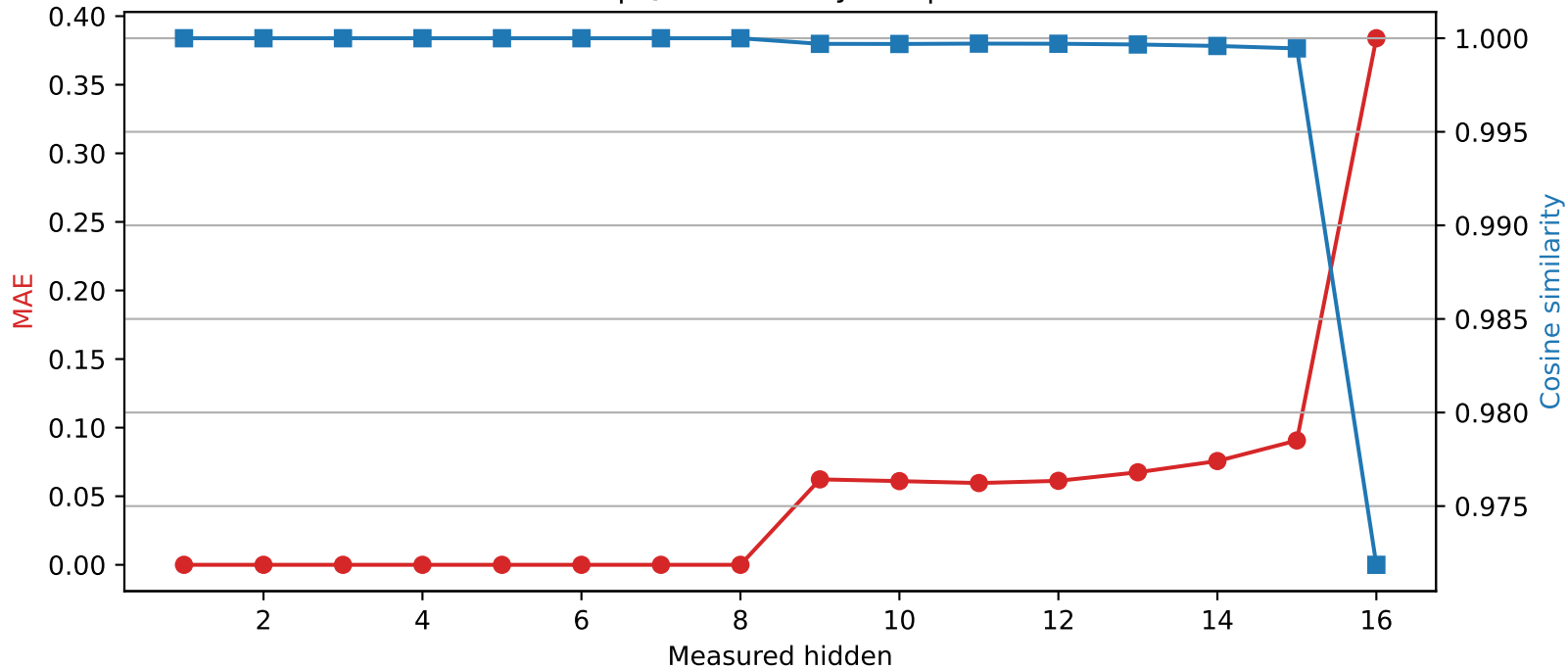
Llama-3.2-1B | Quantized layer 8 | float32 \rightarrow int2
