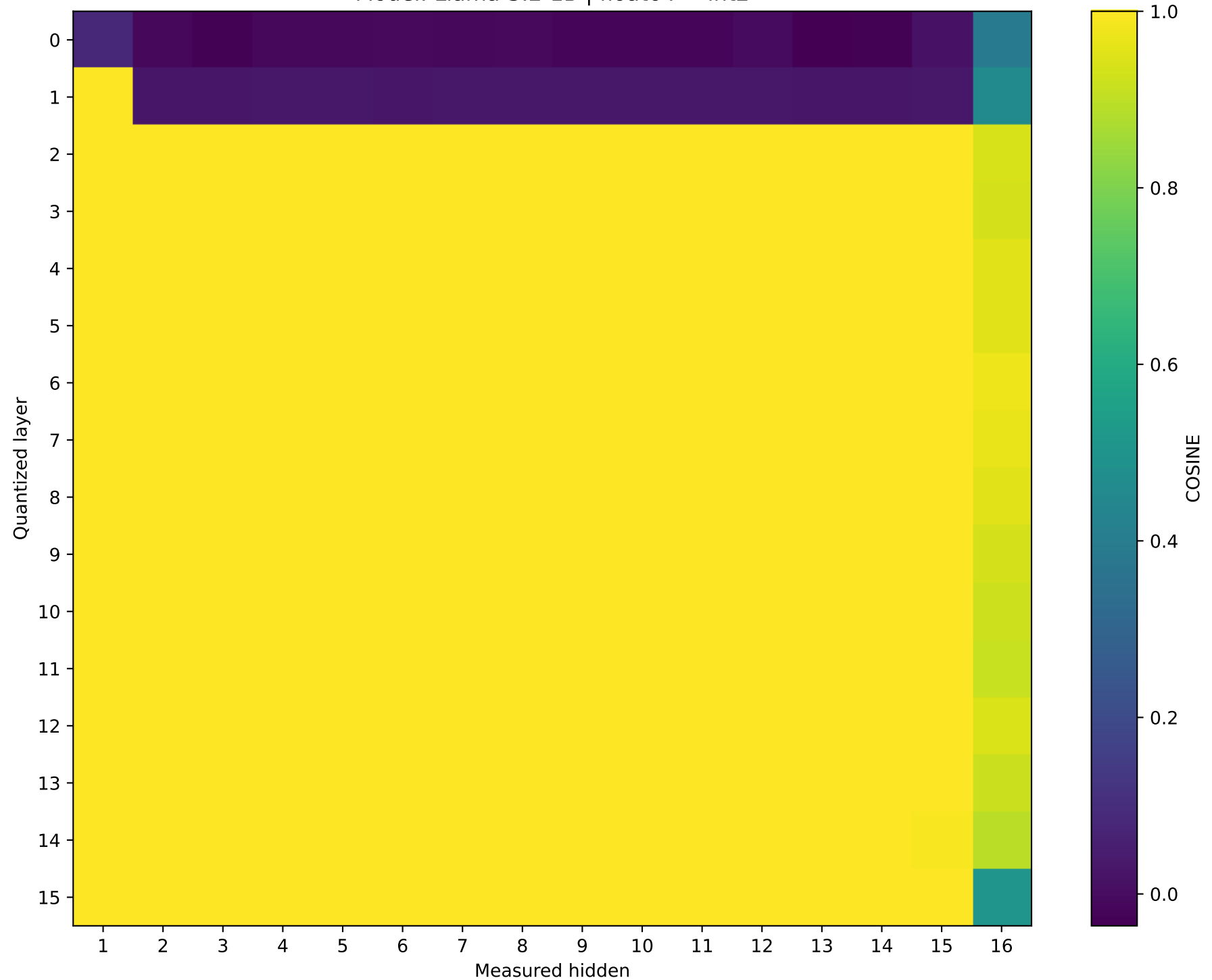
Model: Llama-3.2-1B | float64 → int2
