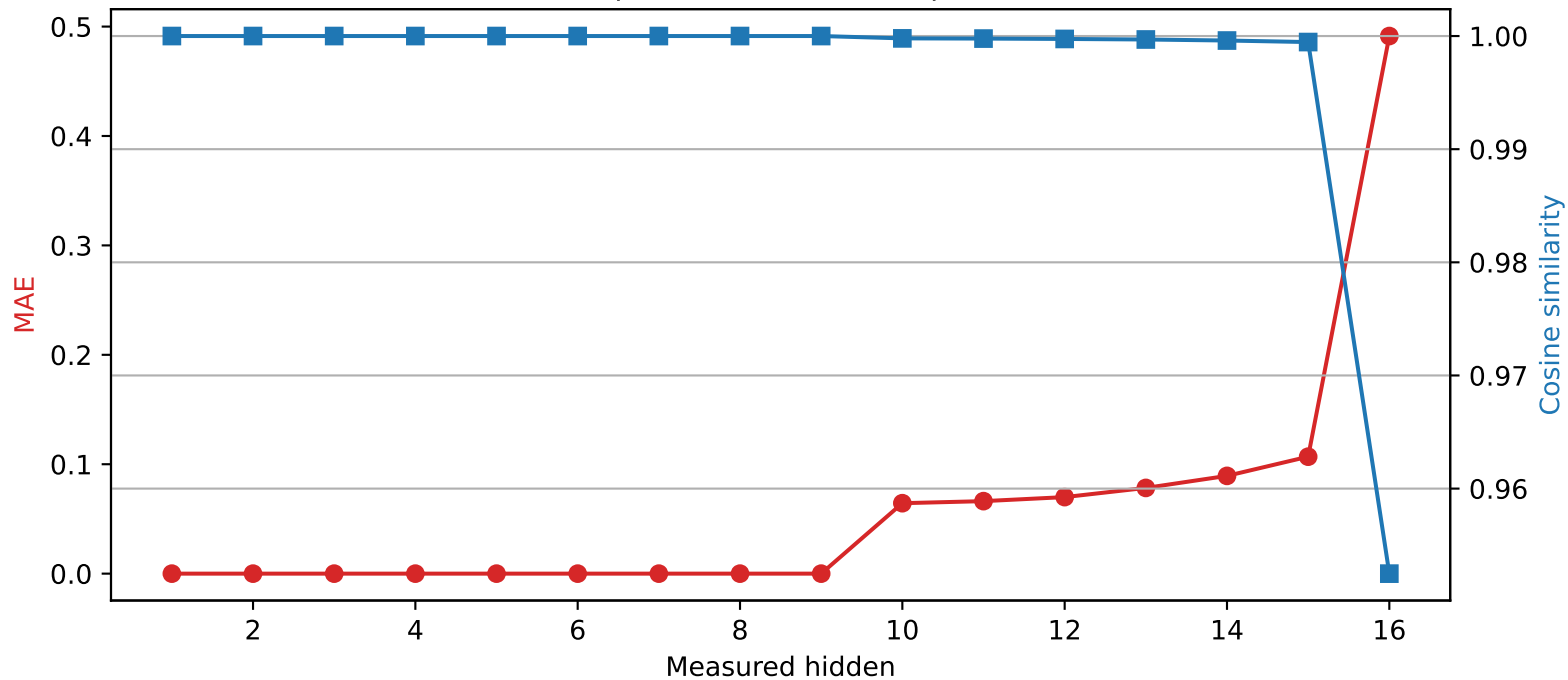
Llama-3.2-1B | Quantized layer 9 | float64 \rightarrow int2
